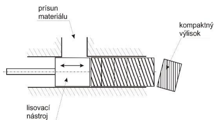
Obrázok 9: Princíp otvorenej lisovacej komory a mechanický kľukový BL 8
